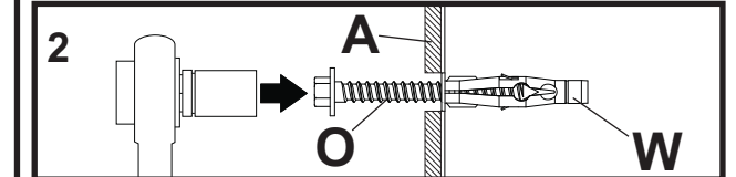
Coloque la placa (A) sobre los anclajes (W) y fijela con los tornillos (O).
